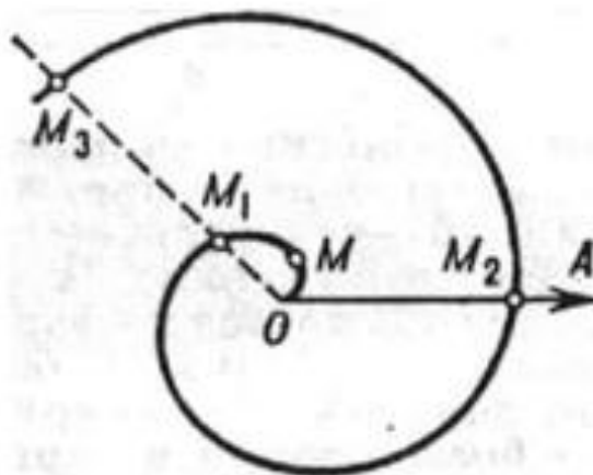
Рис. 3.2. Спираль Архимеда
