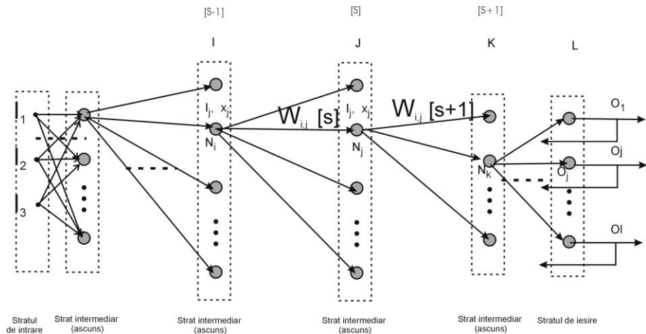
Fig. 3 Arhitectura perceptronului multistrat
