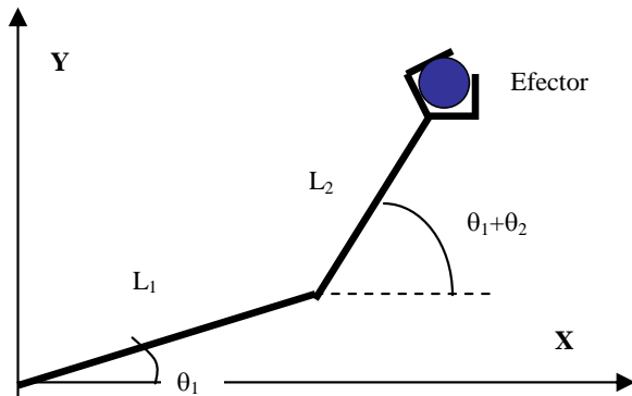
Fig. 4 Structura robotului
