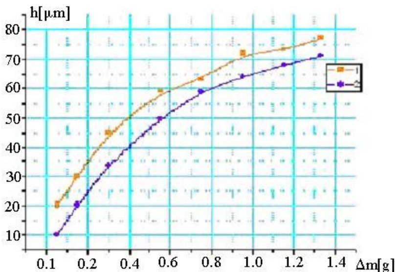
Fig. 2. Grosimea stratului de depunere ca funcție de sporul masei piesei.
