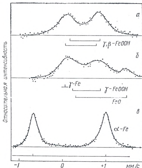
Рис. 1. Мессбауэровские спектры образцов Ст-3 после обработки ИР. Расстояние между электродами 2 (а) и 0,5 мм (б)
