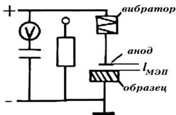
Рис. 1. Схема установки для обработки искровыми разрядами
