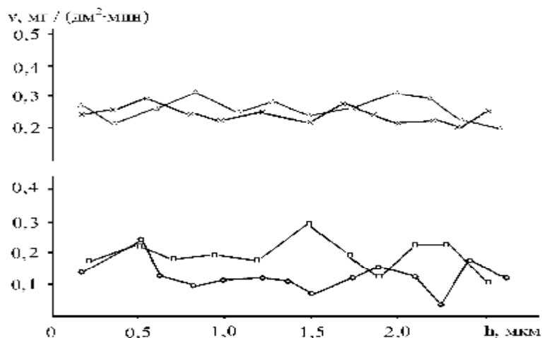
Рис.2. Скорость растворения поверхностных слоев тарного стекла. Продолжительность одного травления 20 мин. X – бутылка (форма 19); \Delta – бутылка (форма 19); P – листовое стекло; O – бутылка (форма 28).
